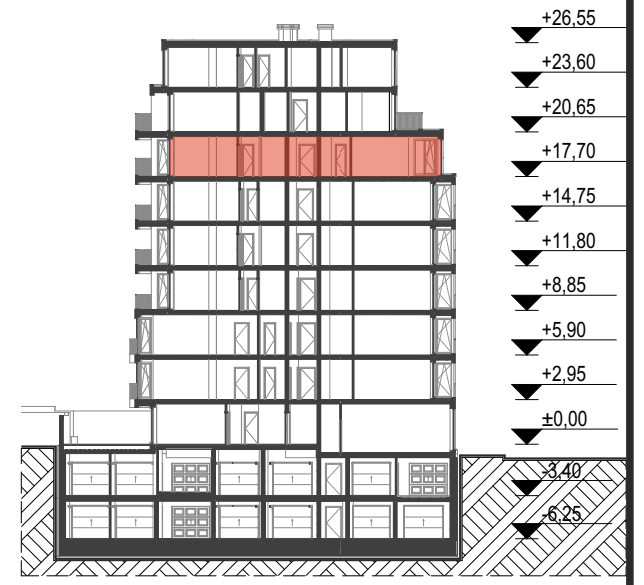
ЗАСТРОЕНИ ПЛОЩИ КОТА +17.70
