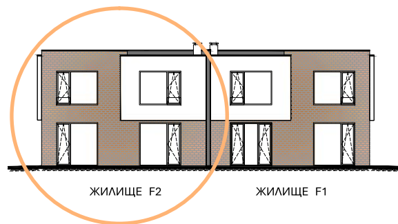
ЖИЛИЩНА ГРУПА F - ФАСАДА ИЗТОК
