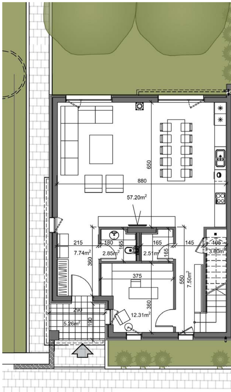
ЖИЛИЩЕ F1 ЕТАЖ 1
