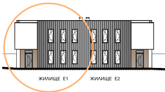
ЖИЛИЩНА ГРУПА E - ФАСАДА ЗАПАД
