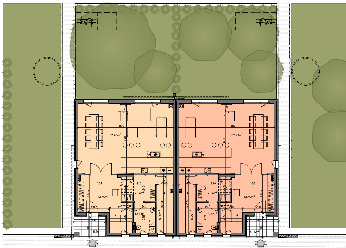
ЖИЛИЩЕ E1 ЕТАЖ 1
