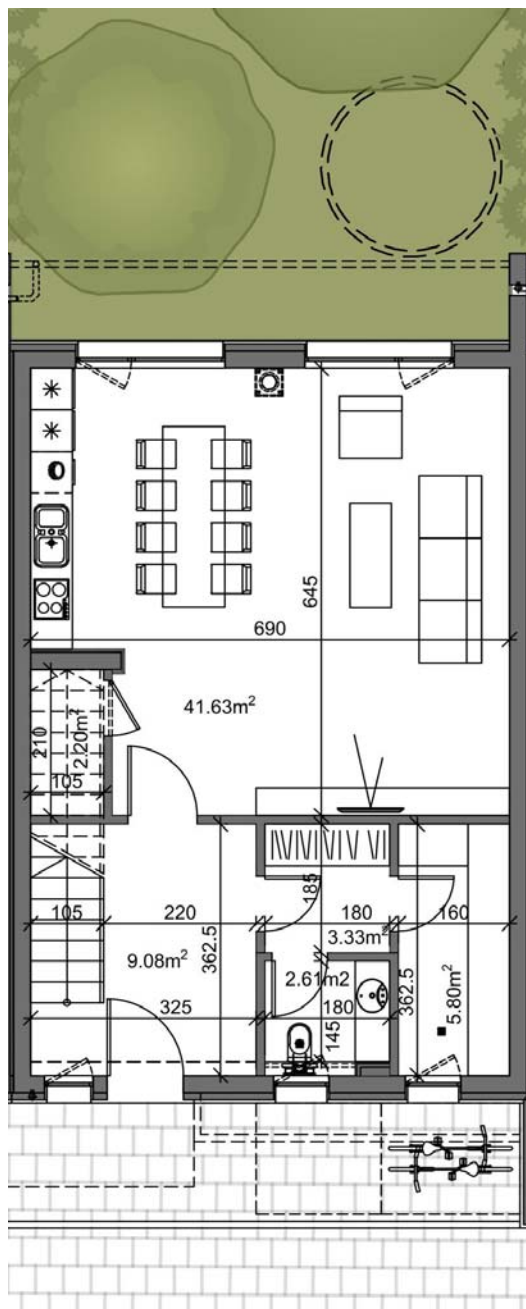
ЖИЛИЩЕ D3 ЕТАЖ 1
