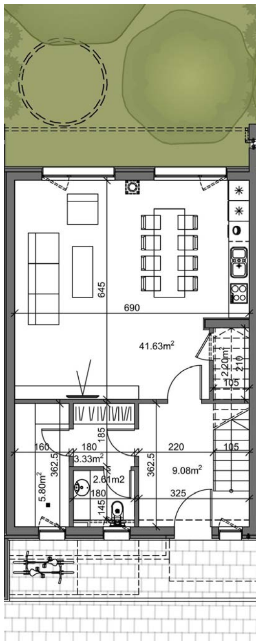
ЖИЛИЩЕ D2 ЕТАЖ 1
