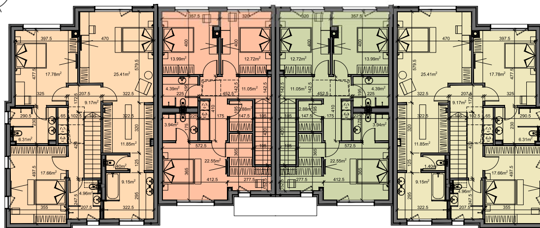
ЖИЛИЩЕ D1 ЕТАЖ 2
