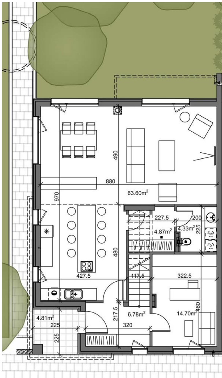
ЖИЛИЩЕ D1 ЕТАЖ 1
