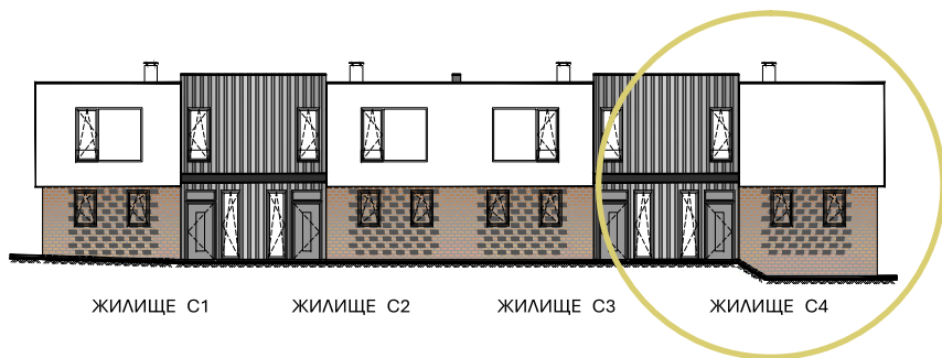
ЖИЛИЩНА ГРУПА С - ФАСАДА ЗАПАД
