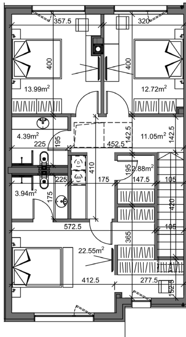
ЖИЛИЩЕ C3 ЕТАЖ 2
