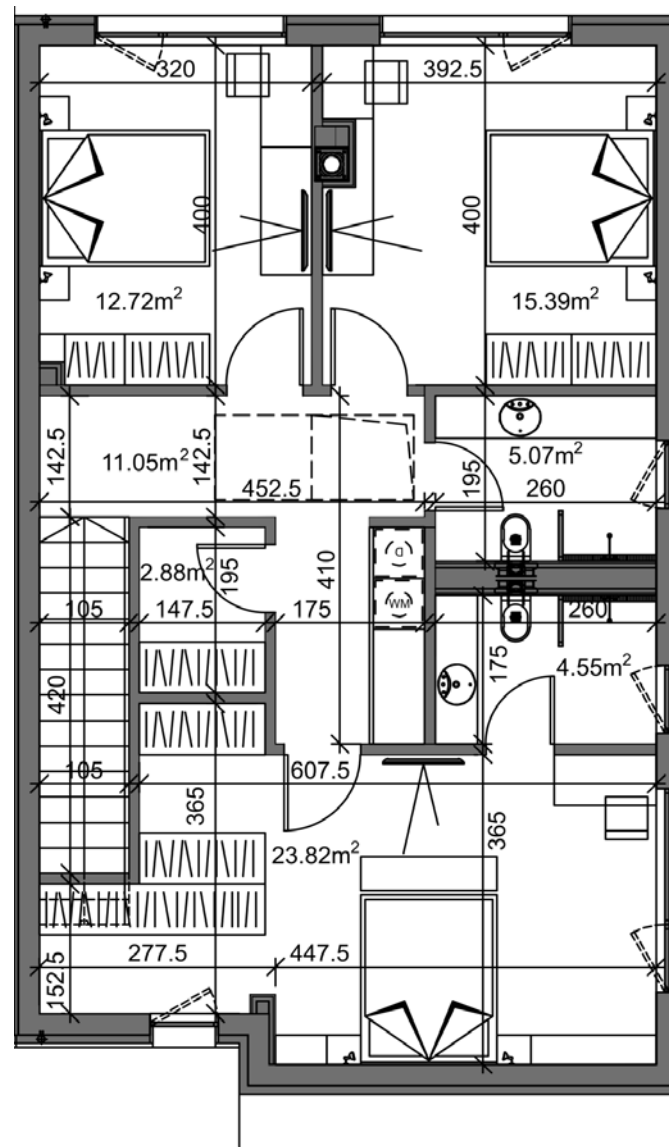
ЖИЛИЩЕ C4 ЕТАЖ 2
