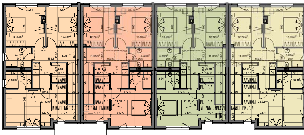
ЖИЛИЩЕ C1 ЕТАЖ 2
