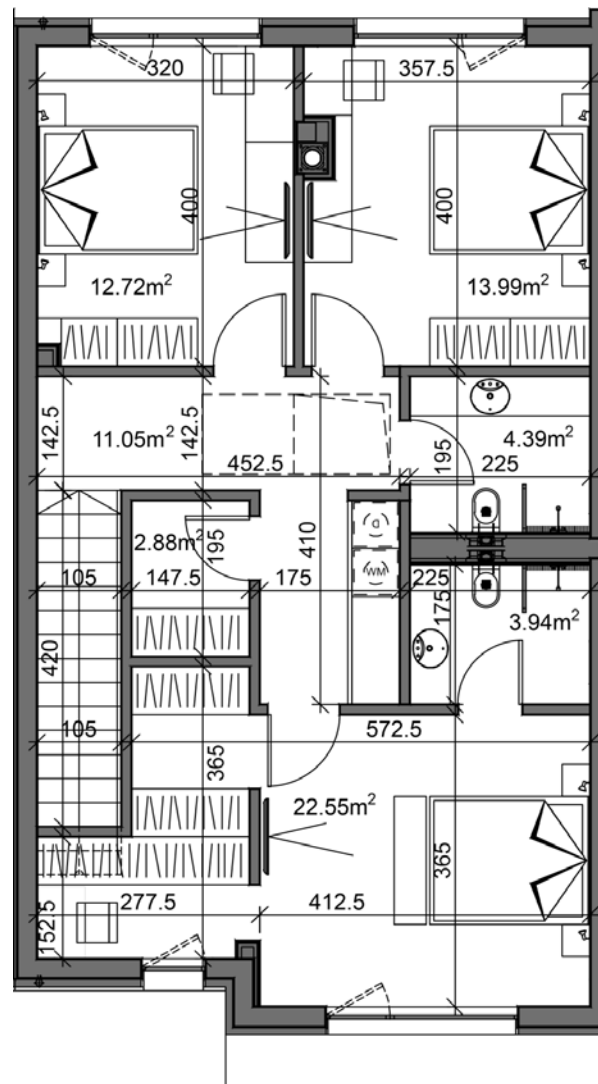
ЖИЛИЩЕ A2 ЕТАЖ 2
