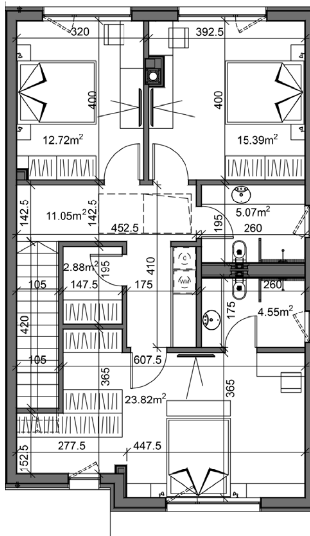
ЖИЛИЩЕ А4 ЕТАЖ 2
