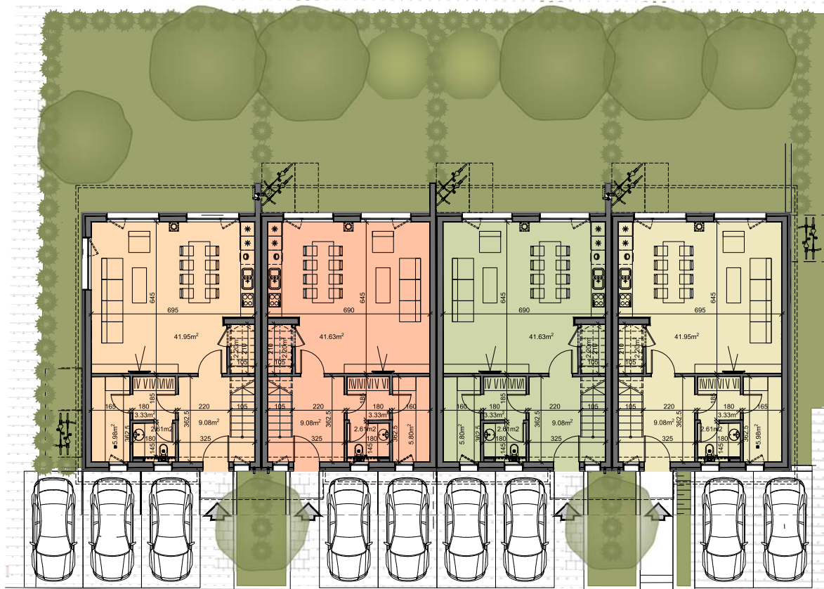
ЖИЛИЩЕ А1 ЕТАЖ 1
