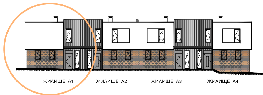
ЖИЛИЩНА ГРУПА А - ФАСАДА ЗАПАД
