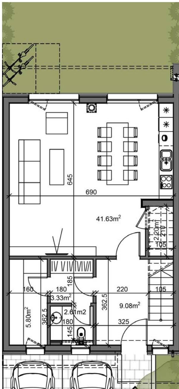
ЖИЛИЩЕ А3 ЕТАЖ 1
