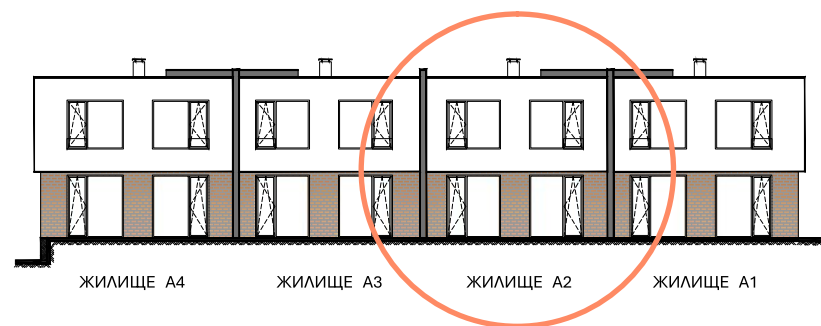
ЖИЛИЩНА ГРУПА А - ФАСАДА ИЗТОК
