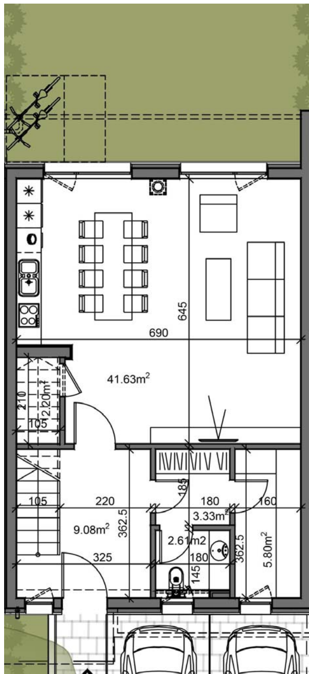
ЖИЛИЩЕ A2 ЕТАЖ 1
