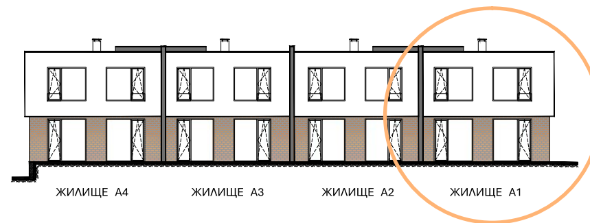
ЖИЛИЩНА ГРУПА А - ФАСАДА ИЗТОК
