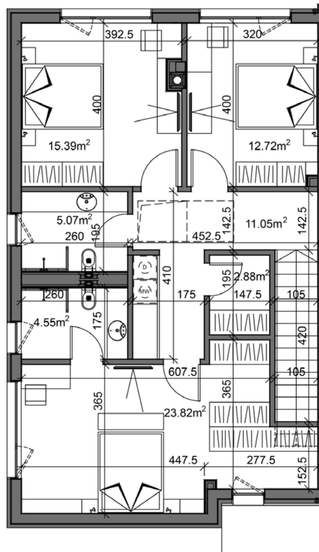
ЖИЛИЩЕ А1 ЕТАЖ 2
